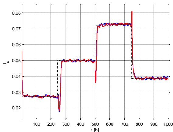
Fig. 3.21 Evoluția criteriului de performanță la optimizare pe baza CRO, considerând că S_{1,in} este cunoscut (albastru) și utilizând estimarea \hat{S}_{1,in} (roșu)
