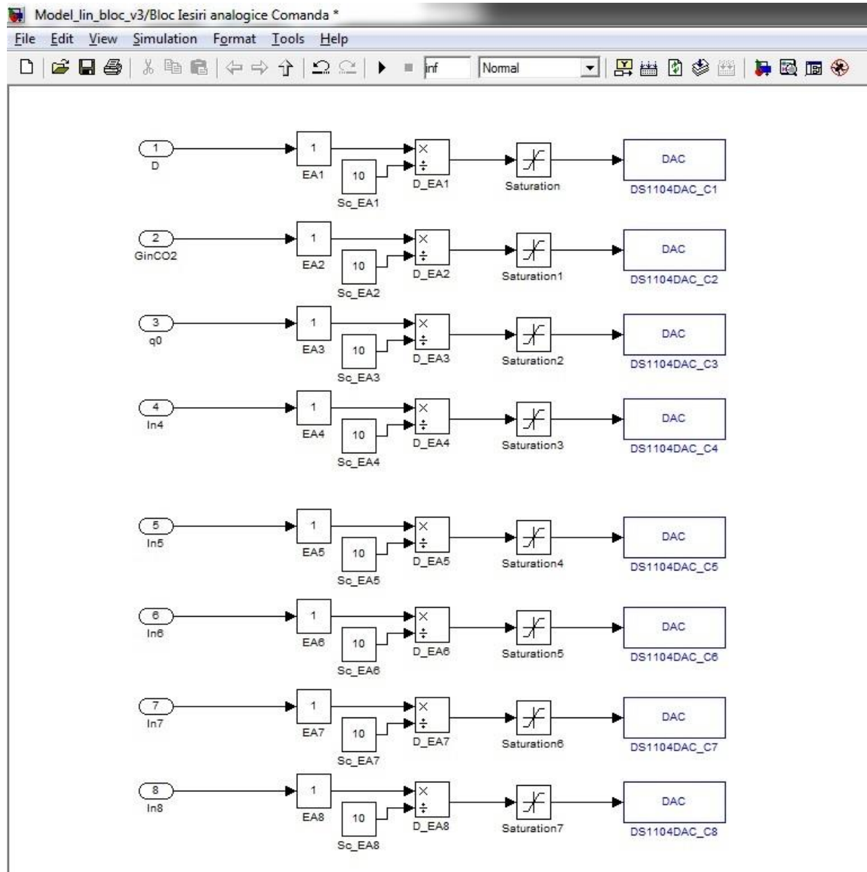
Fig. 2.2d – Modulul de ieșiri analogice
