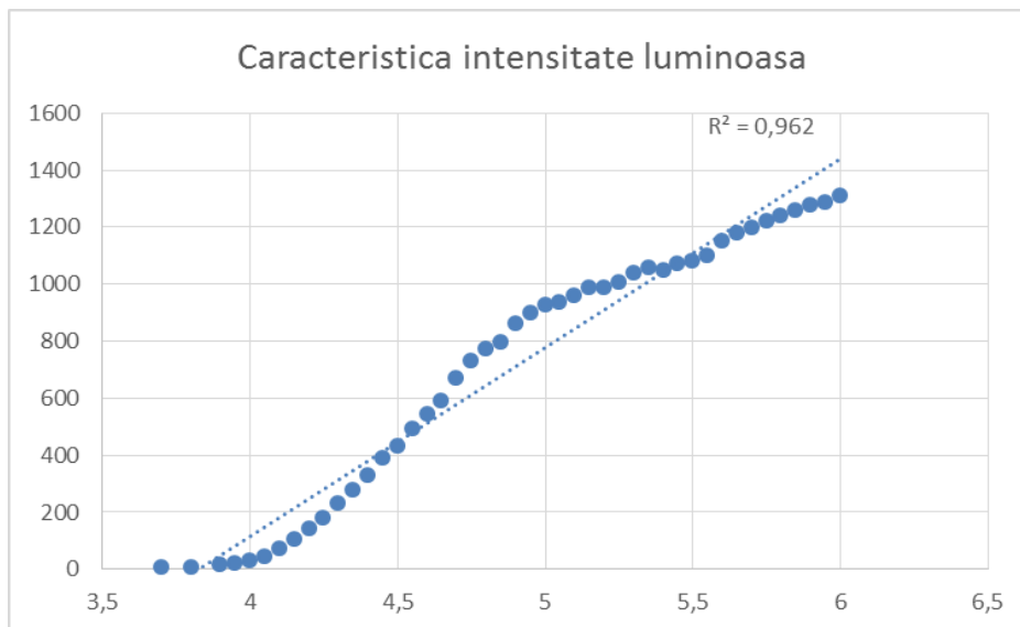
Fig. 7.6 Caracteristica de luminozitate a panoului cu led-uri
