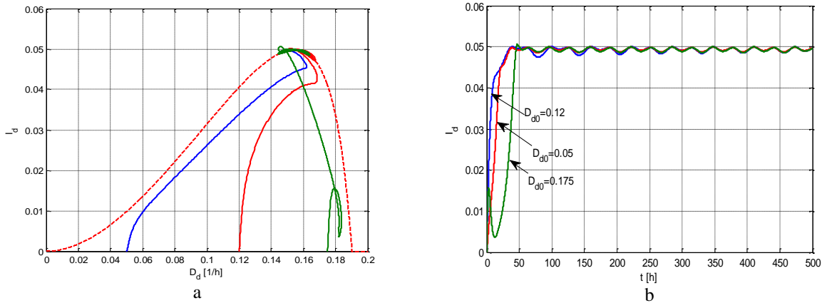
Fig. 3.5 Traiectoria punctului de funcționare în planul D_d-I_b (a) și evoluția criteriului în procesul de optimizare (b), pornind de la diferite valori inițiale ale diluției D_d
