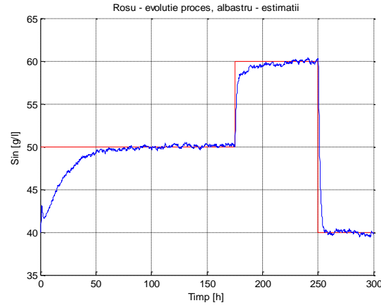
Fig. 3.12 Estimarea parametrului S_{1,in} atunci când acesta are variații în formă de treaptă.
