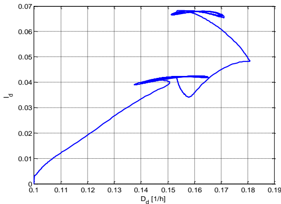
Fig. 3.25 Traiectoria punctului de funcționare în planul D_d-I_b în procesul de optimizare
