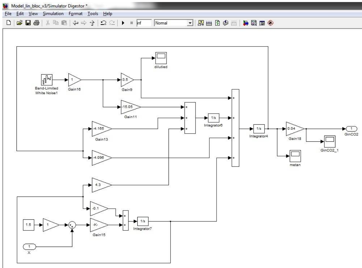
Fig. 2.2e – Modelul digestorului anaerob
