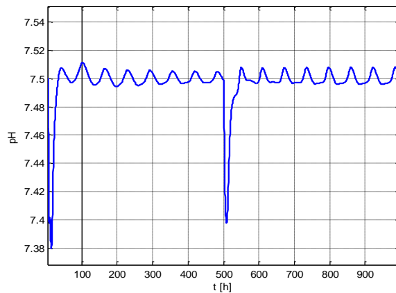
Fig. 3.29 Efectul unei variații în treaptă a concentrației substratului din influxul digesterului, S_{1,in} , asupra pH-ului din PBR
