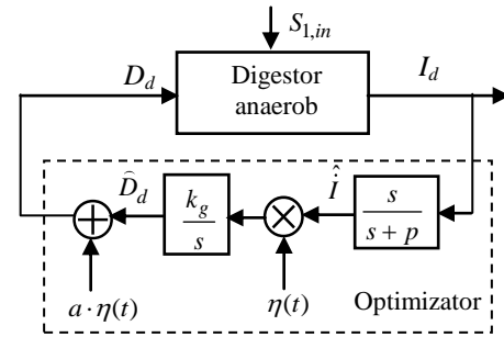
Fig. 3.2 Structura buclei de optimizare a PBR
