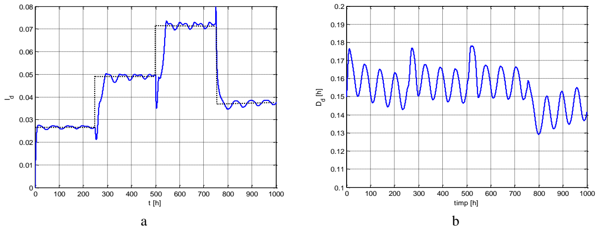
Fig. 3.6 Evoluția criteriului de performanțe (a) și a diluției (b) la variații în treaptă ale perturbației S_{1,in}
