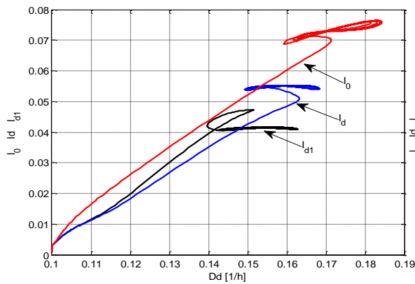
Fig. 3.31 Traiectoriile punctului de funcționare în planul D_d - I_d , în procesul de optimizare, utilizând criteriile de performanță I_0 , I_d și I_{d1}
