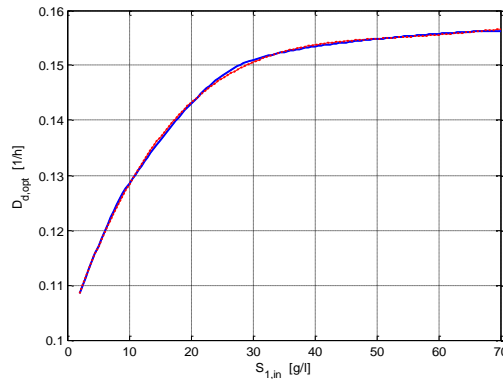
Fig. 3.18 CRO (albastru) și parametrizarea acesteia cu un polinom de gradul 4 (roșu)
