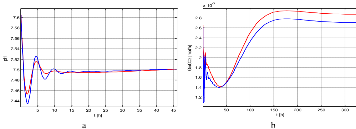
Fig. 3.22 Evoluția pH-ului (a) și a debitului G_{inCO_2} (b) în cadrul buclei de reglare a pH-ului, atunci când nu se consideră (roșu) și când se consideră (albastru) concentrațiile de N 2 și O 2 în gazele arse
