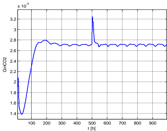
Fig. 3.28 Variația debitului G_{inCO2} [mol/l] (comanda regulatorului de pH) la o variație în treaptă a concentrației substratului în influxul digesterului, S_{1,in}
