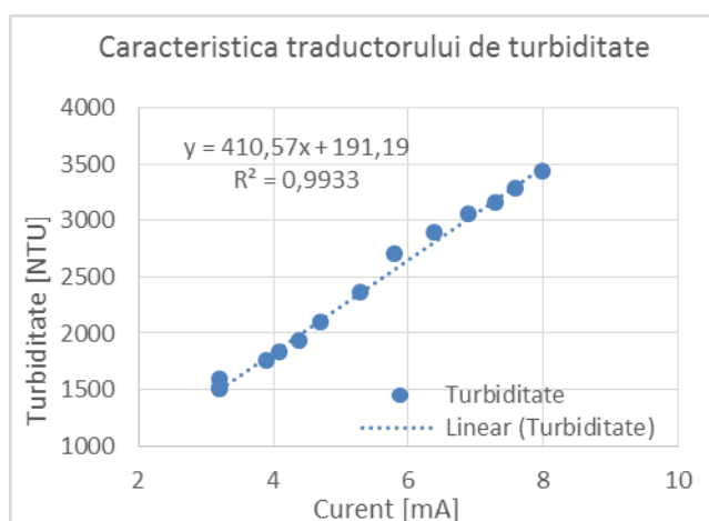
Fig. 7.4 Caracteristica traductorului de turbiditate
