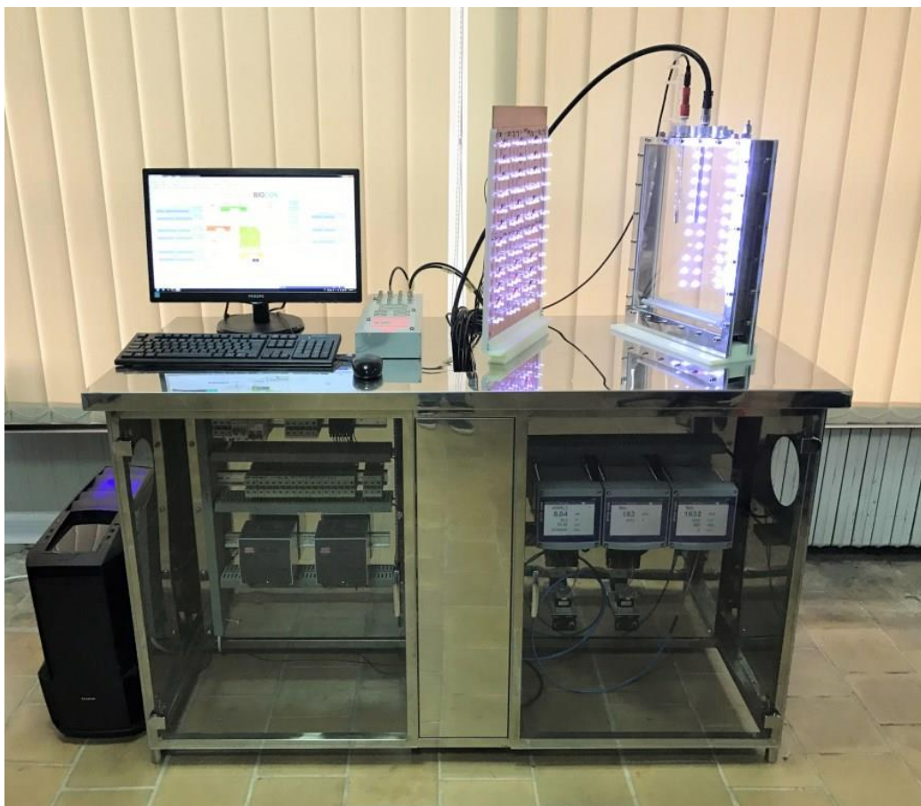
Fig. 1.3 Fotobioreactor cu sistemul de monitorizare si control în funcțiune
