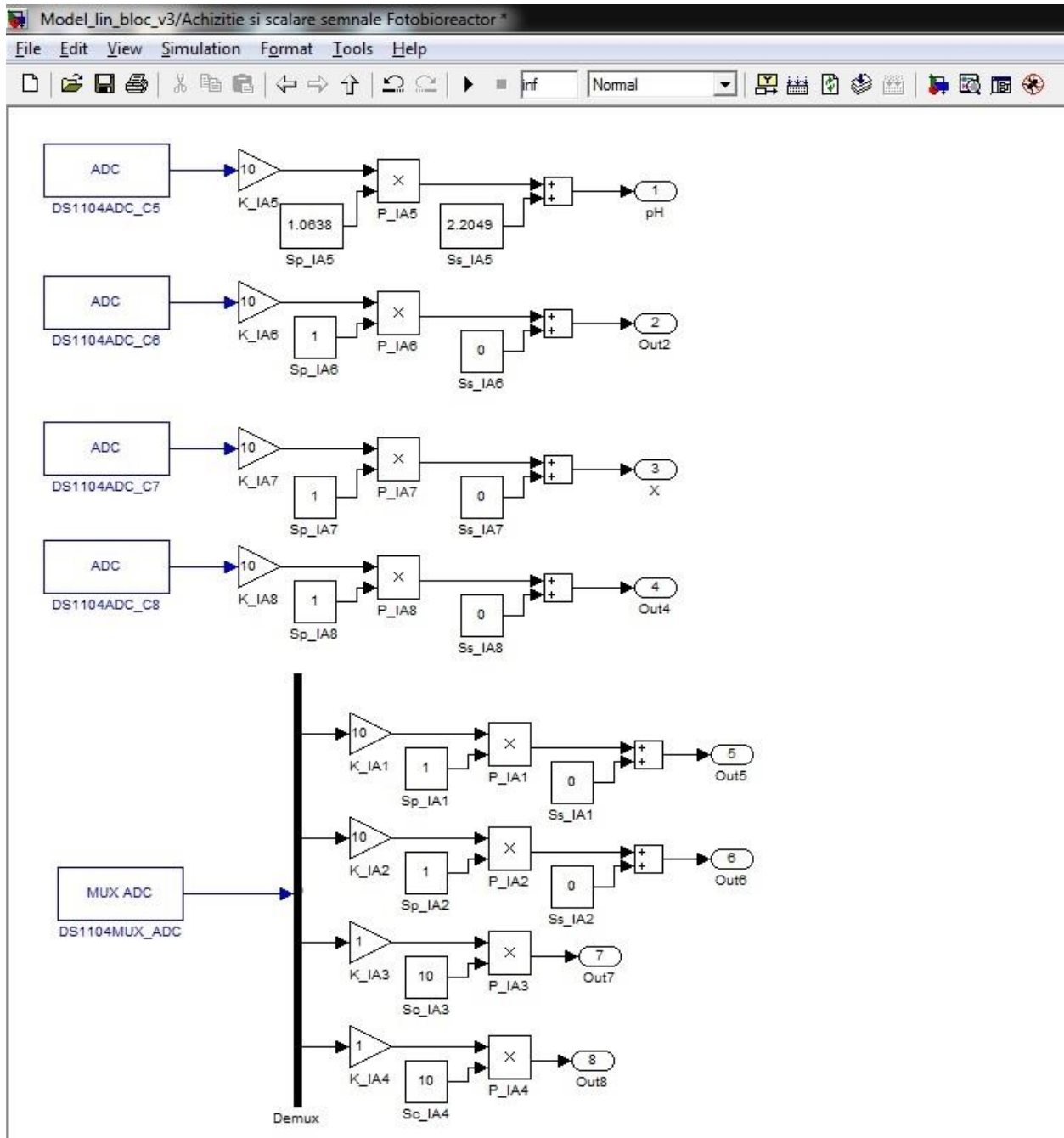
Fig. 2.2b – Modulul de achiziție date și scalare
