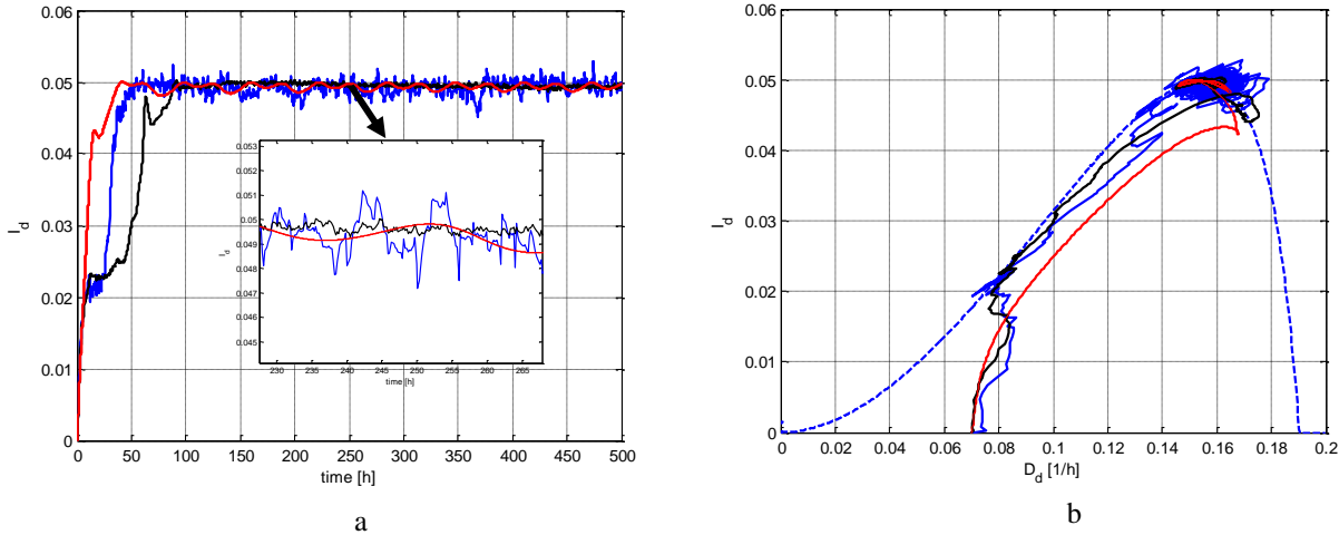
Fig. 3.3 Evoluțiile criteriului I_d (a) și traiectoriile punctului de funcționare în planul D_d - I_d (b) pentru extremum seeking stochastic (albastru), varianta modificată (negru) și varianta deterministă (roșu)
