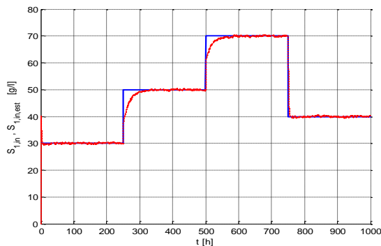
Fig. 3.19 Evoluția variabilei S_{1,in} (albastru) și a estimării \hat{S}_{1,in} (roșu)
