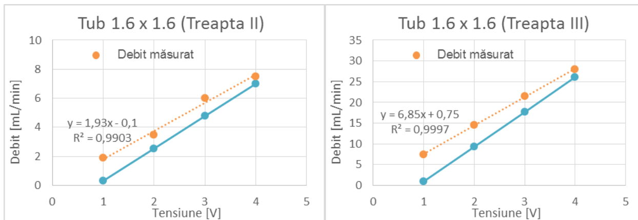
Fig. 7.1 Caracteristici ale pompelor peristaltice Tub 1.6x1.6 (maro – caracteristică reală, albastru – caracteristică de catalog)
