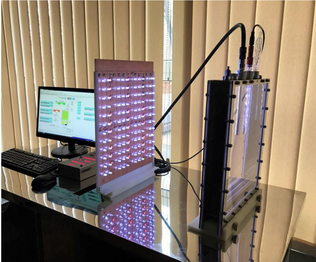
Fig. 5.1 Fotobioreactor comandat de calculator
