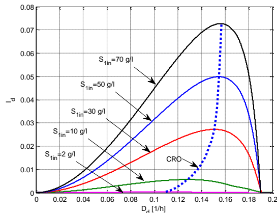
Fig. 3.10 Caracteristica regimurilor optime (CRO) a digesterului
