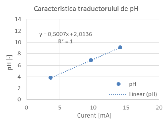
Fig. 7.5 Caracteristica traductorului de pH
