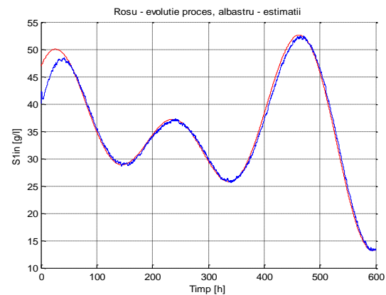
Fig. 3.14 Estimarea parametrului S_{1,in} atunci când acesta are variații de forma unei sume de două sinusoides cu frecvențe diferite
