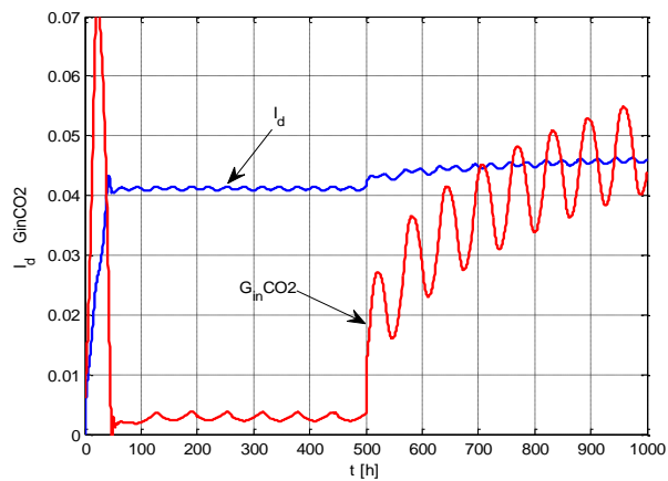
Fig. 3.34 Evoluțiile debitului G_{inCO_2} de la intrarea în PBR și a criteriului I_d de la digester la modificarea referinței regulatorului de pH de la 7.5
