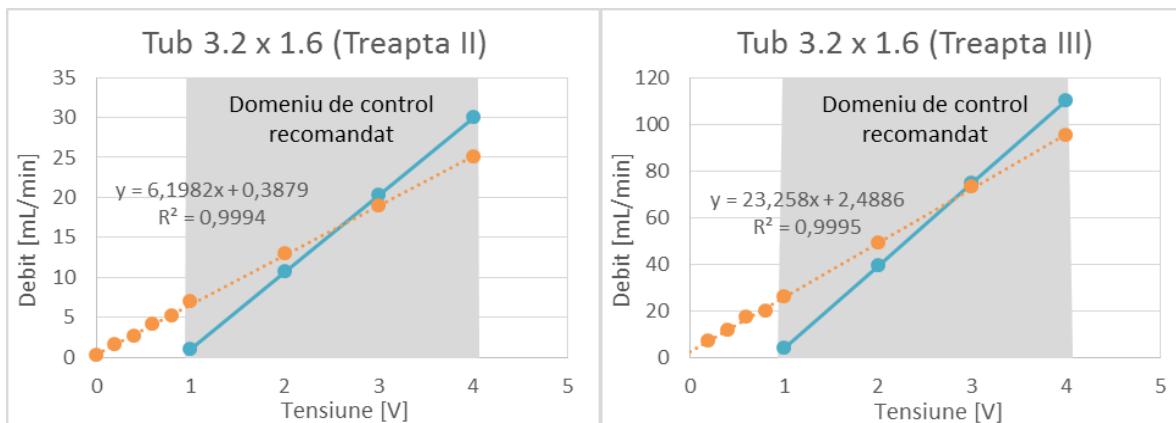
Fig. 7.3 Caracteristici ale pompelor peristaltice Tub 3.2x1.6, Trapta 3 (maro – caracteristică reală, albastru – caracteristică de catalog)
