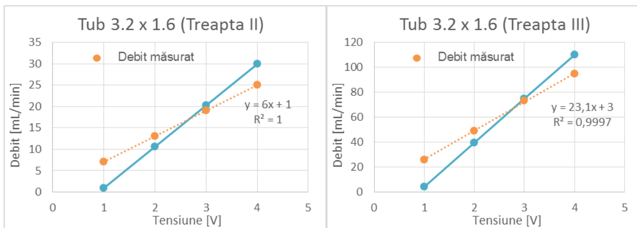
Fig. 7.2 Caracteristici ale pompelor peristaltice Tub 3.2x1.6 (maro – caracteristică reală, albastru – caracteristică de catalog)
