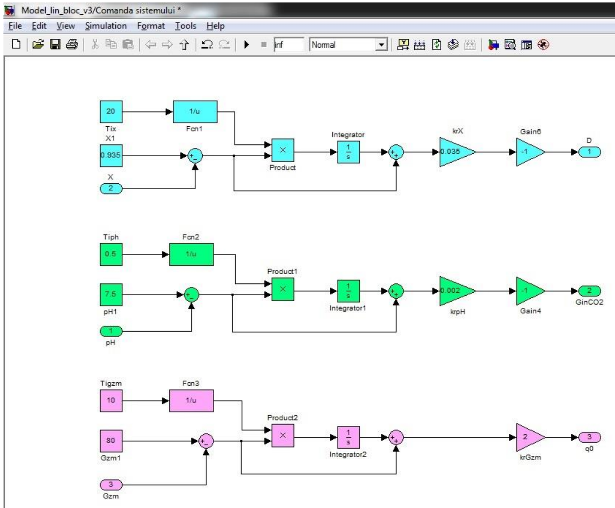
Fig. 2.2c – Modulul reguletoarelor pentru cele trei bucle (biomasă, pH și intensitate luminoasă)
