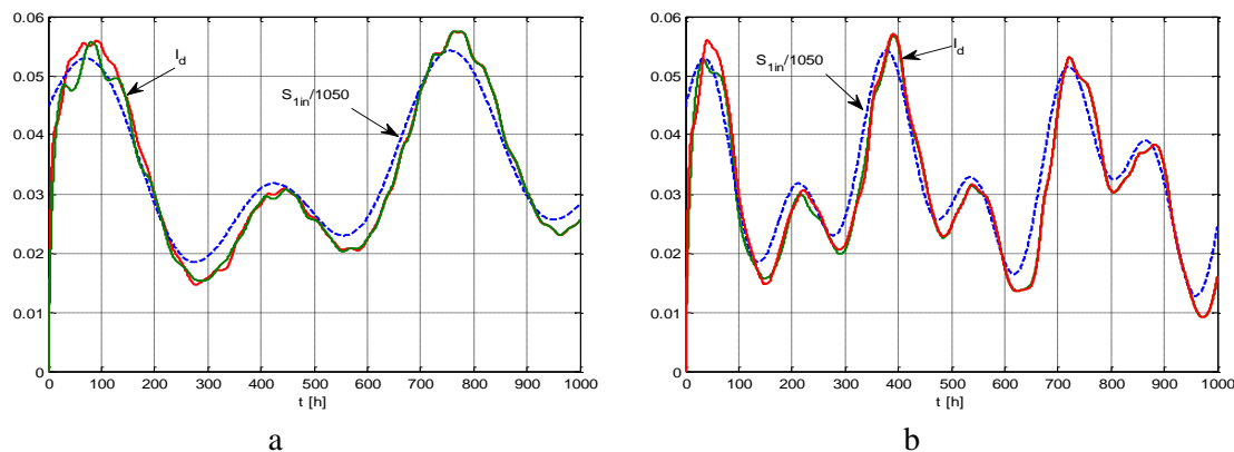
Fig. 3.8 Evoluțiile criteriului de performanță pentru D_{d0} = 0.01 [g/l] (roșu) și D_{d0} = 0.1 [g/l] (negru), atunci când mărimea perturbatoare S_{1,in} (albastru), are forma (6), cu valorile indicate ale pulsațiilor \omega_1 și \omega_2 (a) și când valorile acestor pulsații se dublează (b) în care \omega_1 = 0.0375 / 2 [rad/s] și \omega_2 = (0.0375 \cdot \sqrt{0.2}) / 2 [rad/s].
