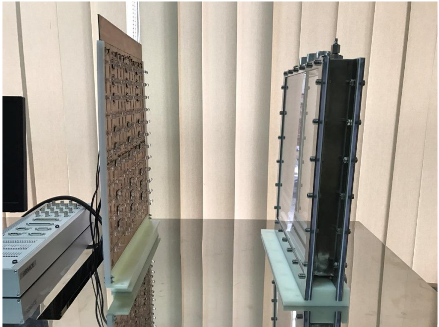
Fig. 1.2 Fotobioreactor și panou cu leduri
