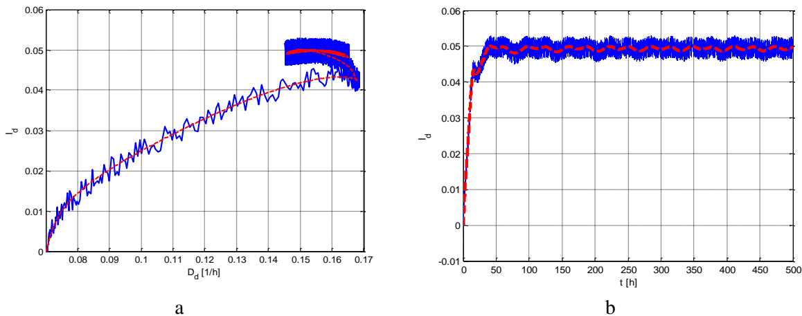
Fig. 3.9 Traiectoria de optimizare în planul D_d - I_d (a) și evoluția criteriului de performanță (b) în prezența zgomotului adițional la ieșire
