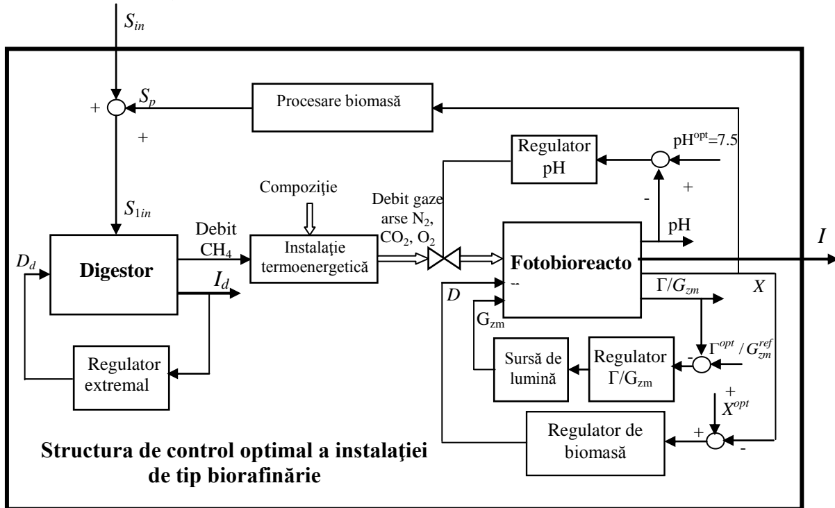
Fig. 3.27 Schema de control optimal al instalației de tip biorafinării, pe baza soluțiilor de optimizare a digesterului și fotobioreactorului
