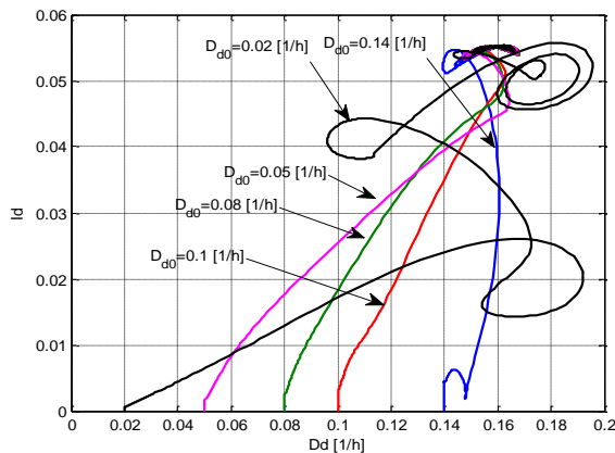
Fig. 3.23 Traiectoriile punctului de funcționare în planul D_d-I_b , în procesul de optimizare, pornind de la diferite valori inițiale ale diluției D_{d0}
