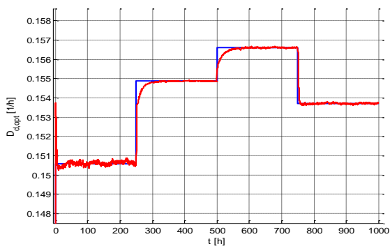
Fig. 3.20 Evoluția diluției optime la utilizarea variabilei S_{1,in} (albastru) și la utilizarea estimării \hat{S}_{1,in} (roșu)
